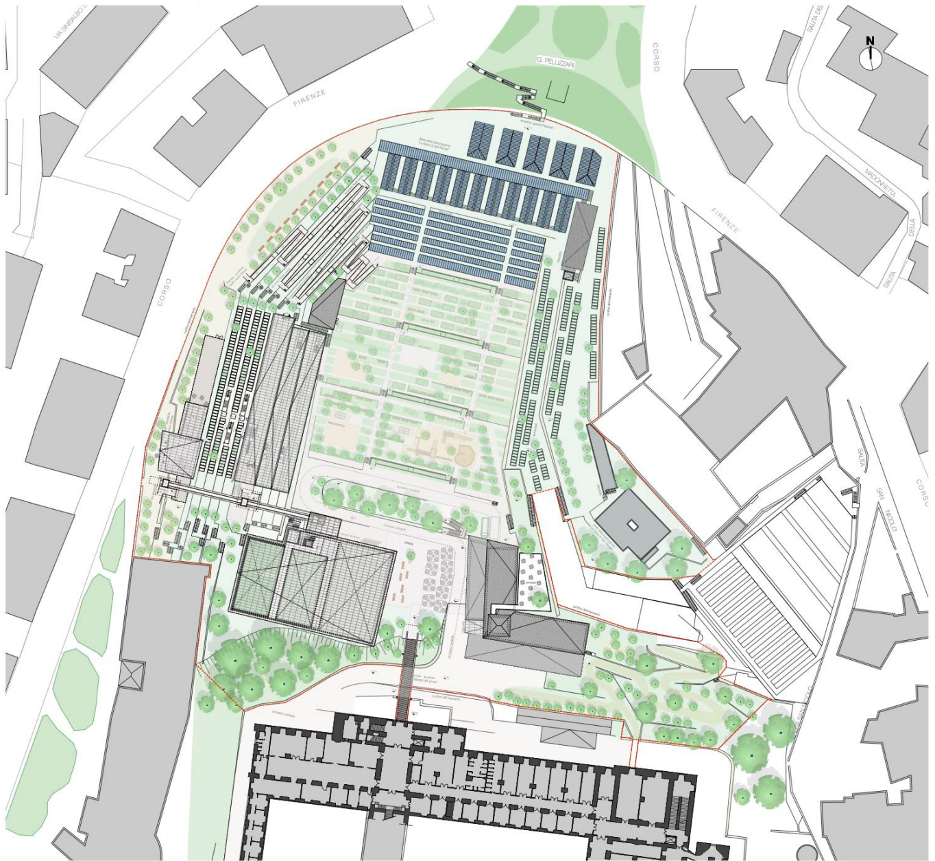
pianimetria generale Scale: 1:500
