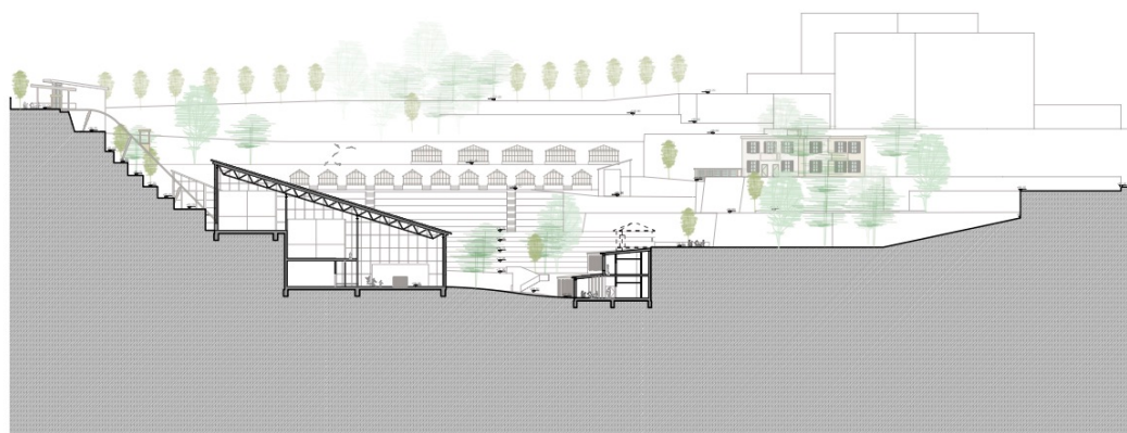
sezione BB Scale: 1:500
